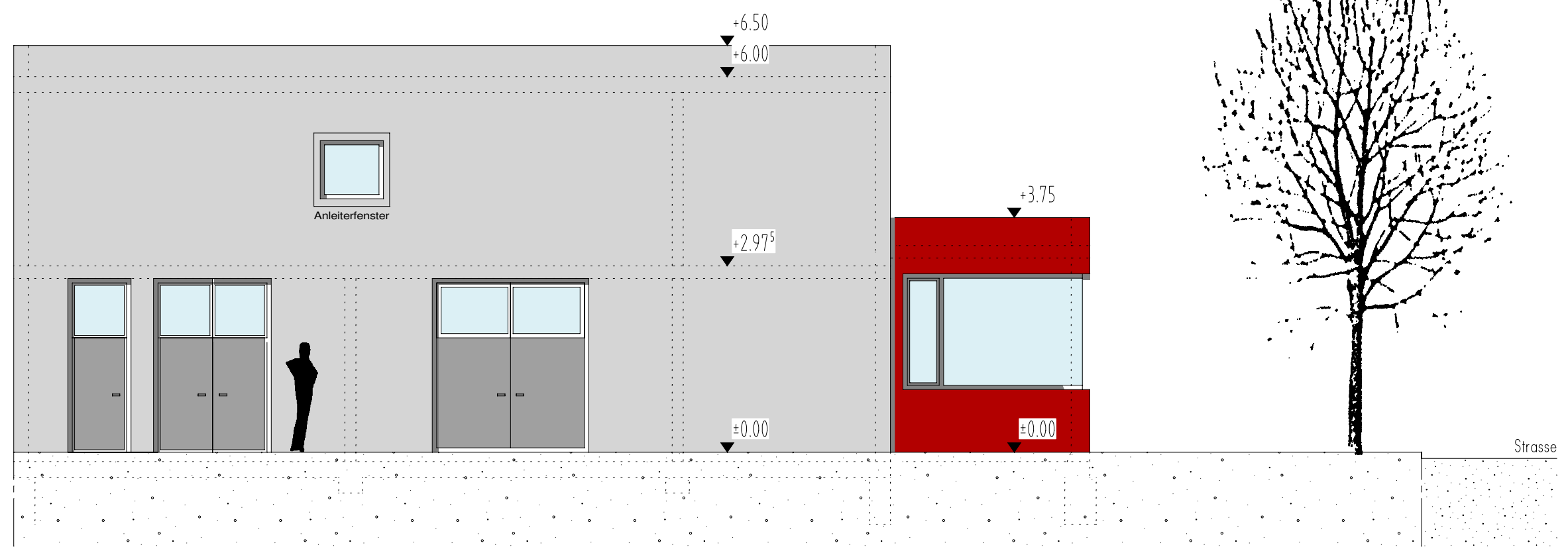
Ansicht Süd
